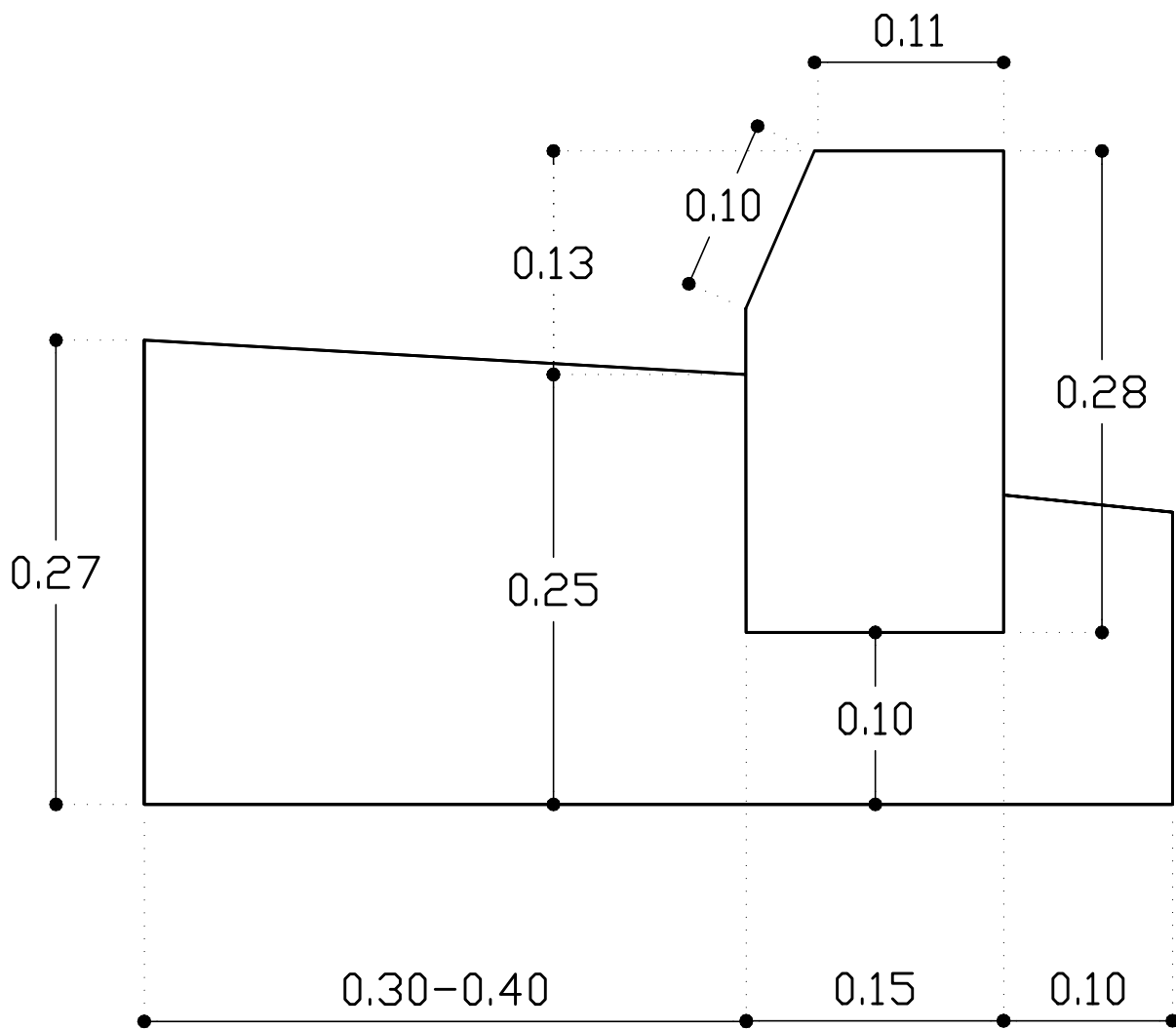
ΛΕΠΤΟΜΕΡΕΙΑ ΚΡΑΣΠΕΔΟΡΕΙΥΡΟΥ ΚΛΙΜ. 1:10
