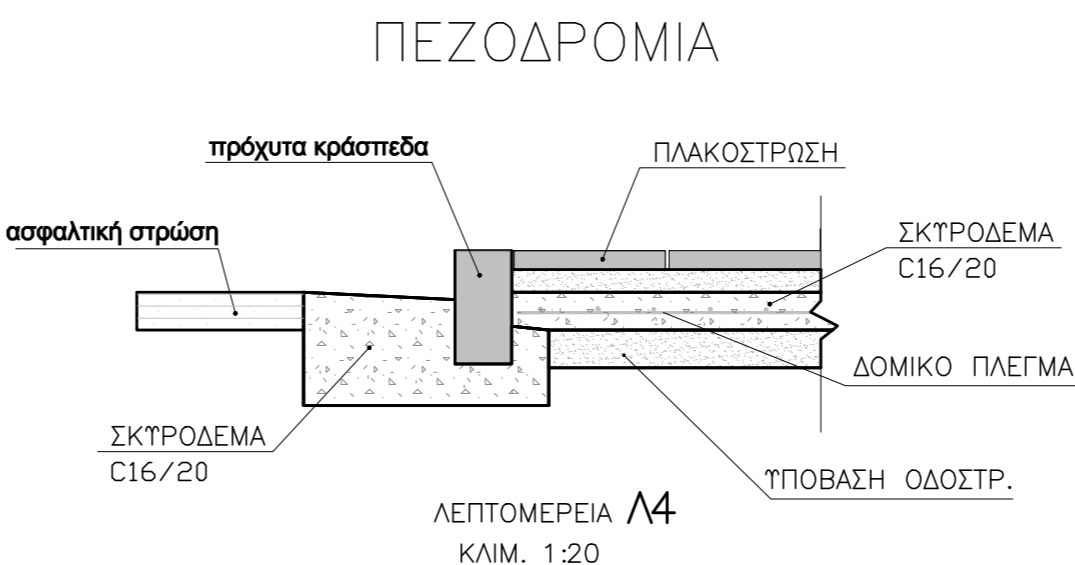
ΛΕΠΤΟΜΕΡΕΙΑ ΚΛΙΜ. 1:20
