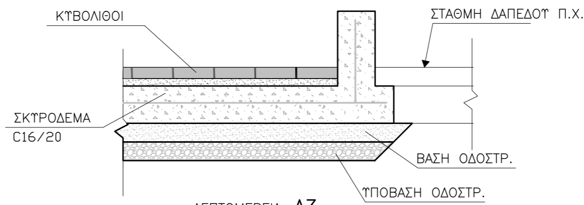
ΛΕΠΤΟΜΕΡΕΙΑ ΚΛΙΜ. 1:20
