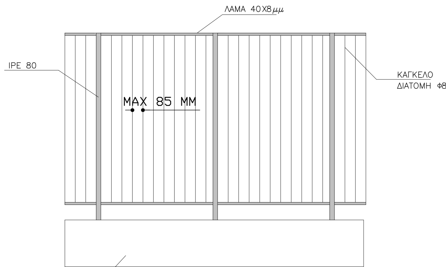
ΕΝΔΕΙΚΤΙΚΗ ΛΕΠΤΟΜΕΡΕΙΑ ΜΕΤΑΛΛΙΚΗΣ ΠΕΡΙΦΡΑΣΗΣ ΚΛΙΜ. 1:20
