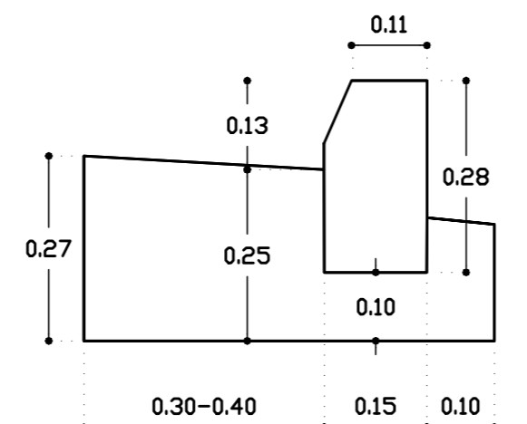
ΛΕΠΤΟΜΕΡΕΙΑ ΚΡΑΣΠΕΔΟΡΕΥΤΡΟΥ ΚΛΙΜ. 1:10
