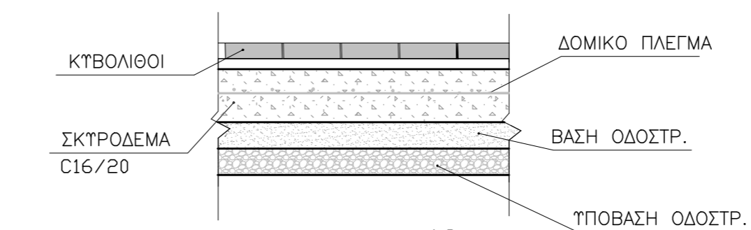
ΛΕΠΤΟΜΕΡΕΙΑ ΚΛΙΜ. 1:20
