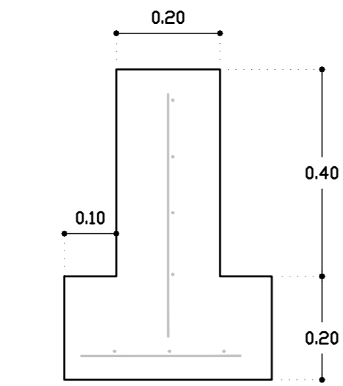
ΛΕΠΤΟΜΕΡΕΙΑ ΤΟΙΧΕΙΟΥ ΚΛΙΜ. 1:10
