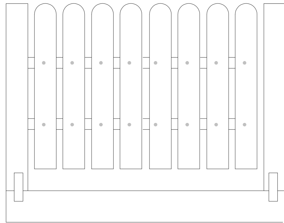
ΕΝΔΕΙΚΤΙΚΗ ΛΕΠΤΟΜΕΡΕΙΑ ΞΥΛΙΝΗΣ ΠΕΡΙΦΡΑΣΗΣ ΚΛΙΜ. 1:10
